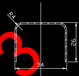
工件图
