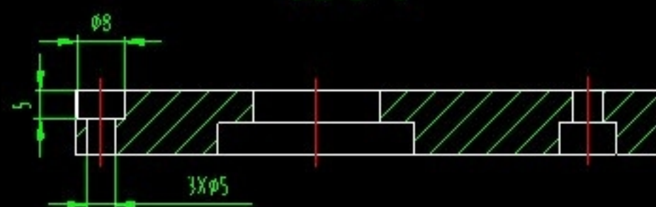
剖面 B-B
