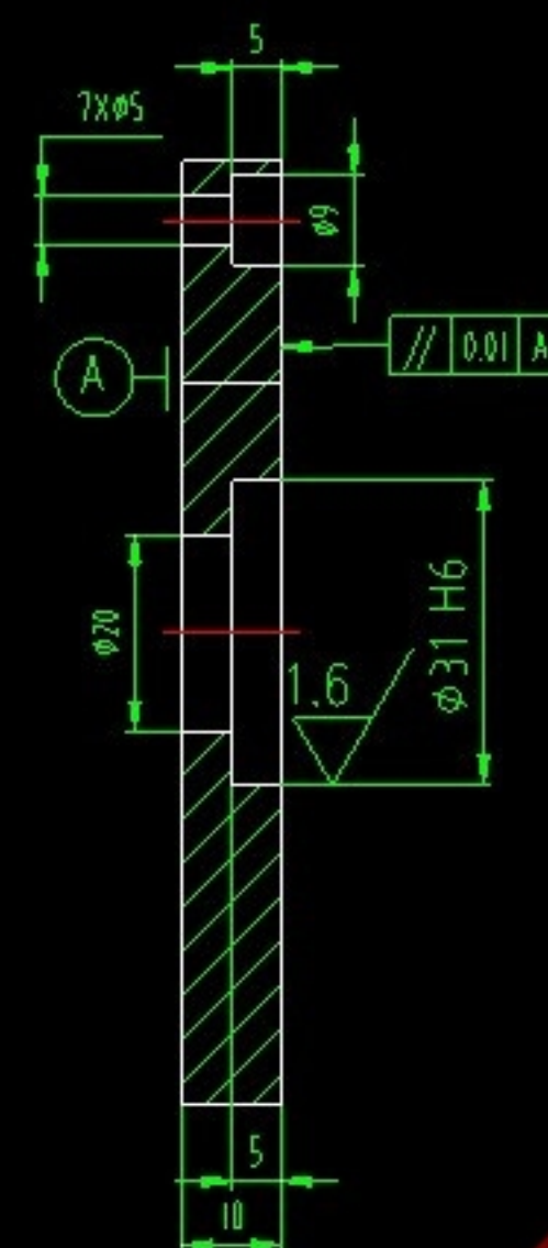
剖面 A-A
