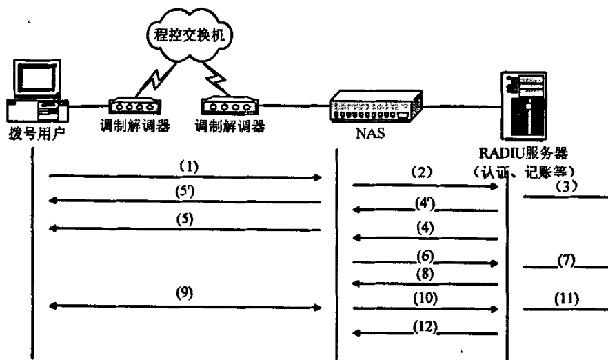
图 3.15 RADIUS 工作流程图
