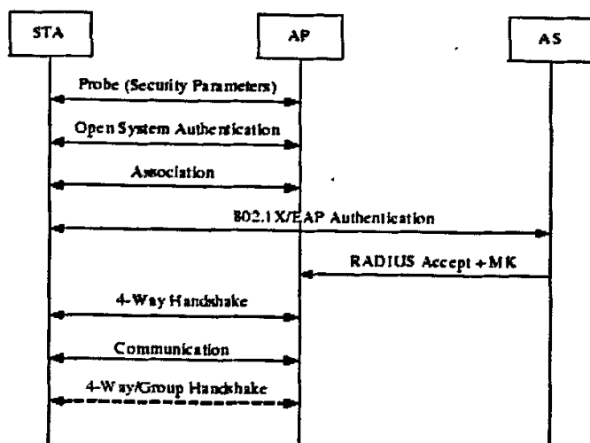
图 3.17 802.11i 完整接入流程
