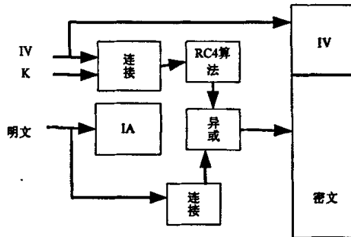
图 2.1 WEP 机制加密原理
