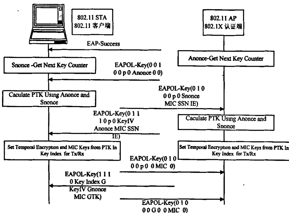
图 3.16 密钥初始化
