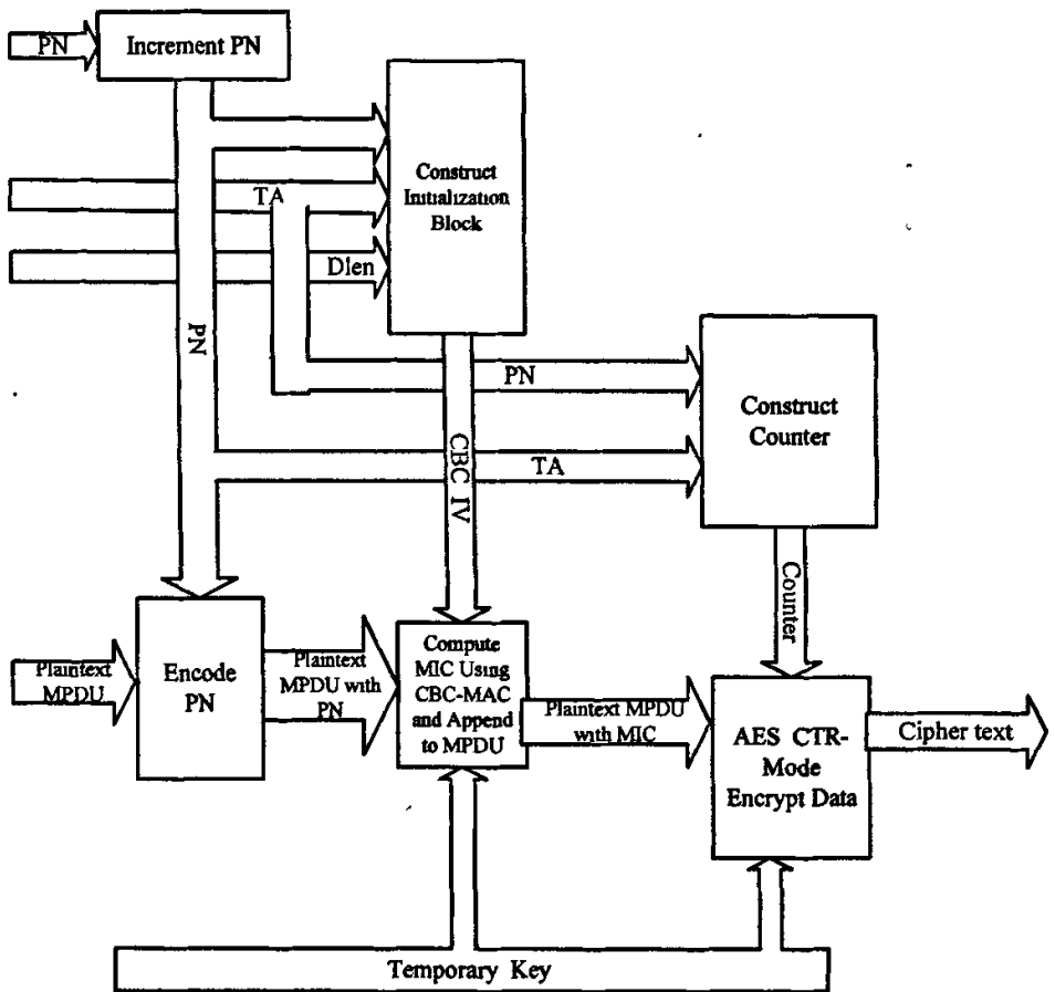
图 3.3 CCMP 加密方块图
