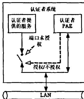
图 3.6 受控和非受控端口
