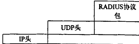
图 3.13 RADIUS 报文格式
