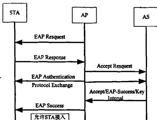
图 3.9 EAP 认证过程简图
