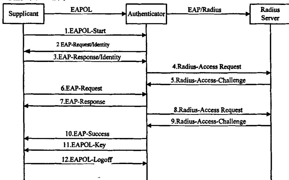
图 3.8 802.1X 认证过程
