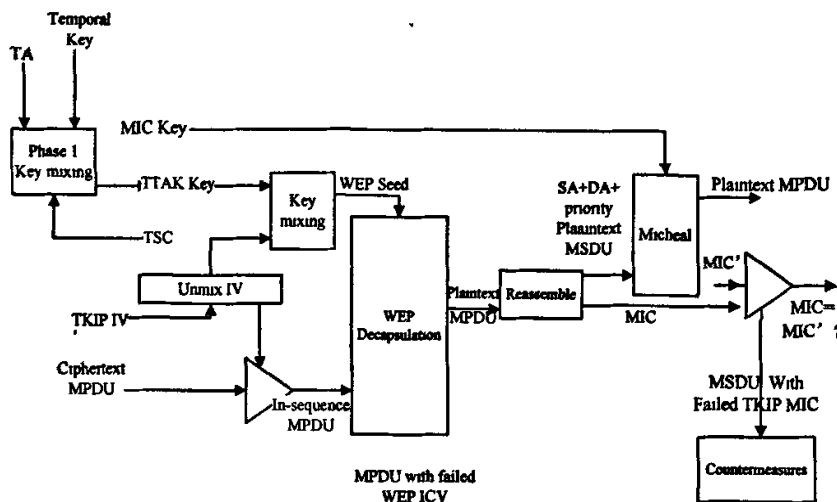
图 3.2 TKIP 解密方块图
