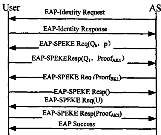
图 5.1 EAP-SPEKE 协议流程
