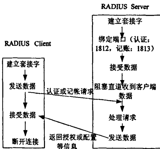
图 3.12 RADIUS 协议通讯过程
