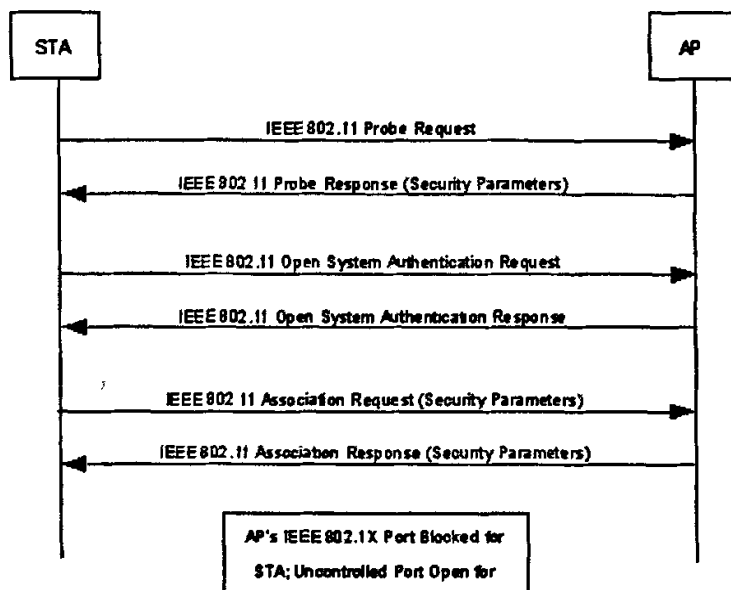
图 3.7 802.1X 认证前接入过程
