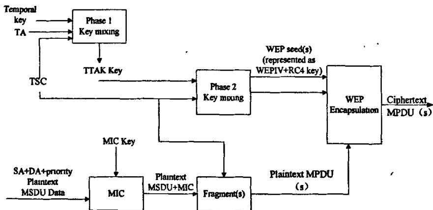
图 3.1 TKIP 加密方块图
