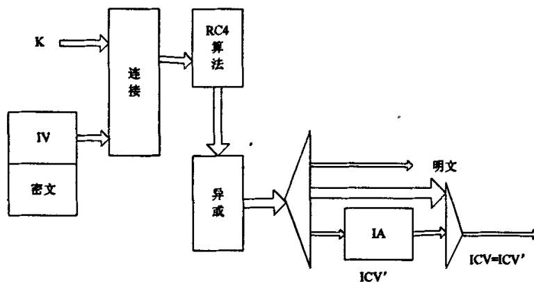
图 2.2 WEP 机制解密原理
