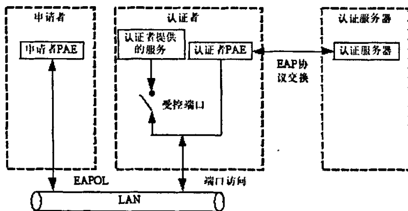
图 3.5 802.1X 体系结构
