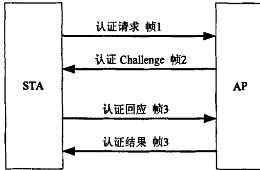
图 2.3 共享密钥认证
