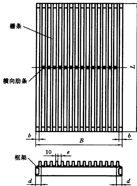
图 1 A 型平面格栅
