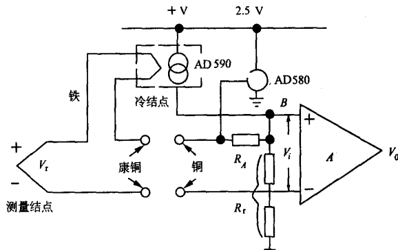
图 3 热电偶的冷端温度补偿
