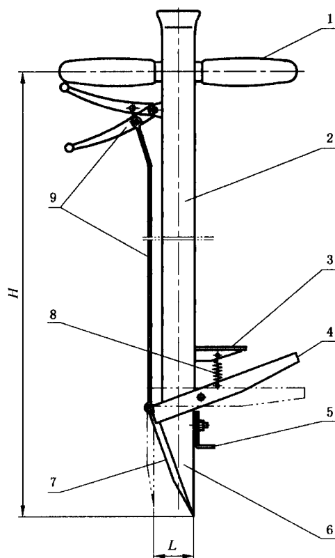
图 1 容器苗栽植器结构示意图
