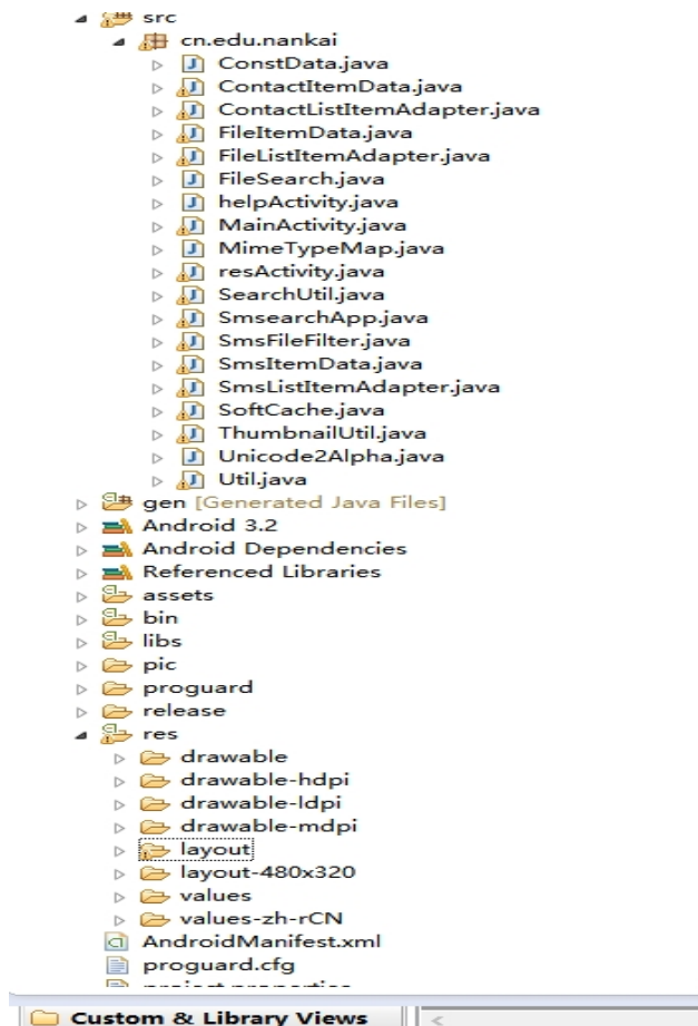
图 5.1 AnySearch 源代码结构图
