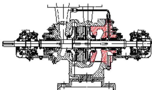
(六) 两级双吸两端支承式离心油泵结构图
