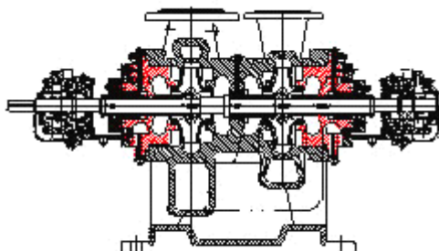
(六) 两级双吸两端支承式离心油泵结构图
