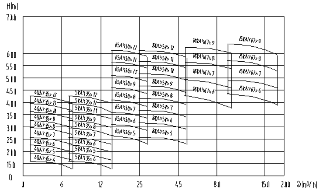
AY 型多级油泵型谱图
