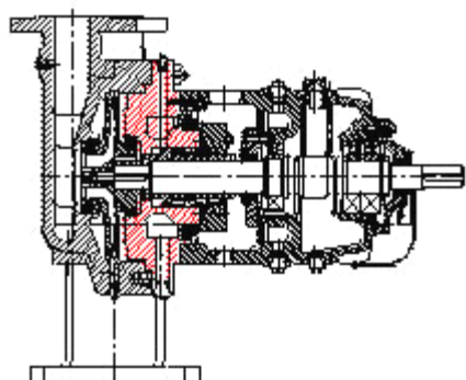
(三) 两级单吸悬臂式离心油泵结构图
