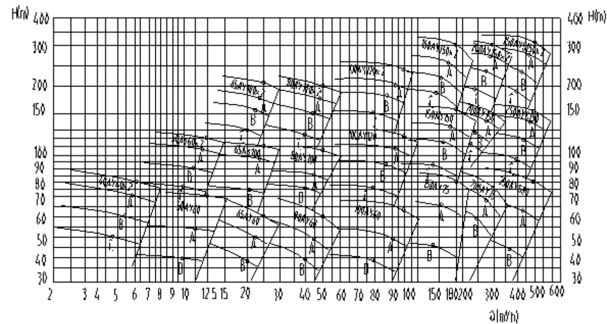
AY 型多级油泵型谱图
