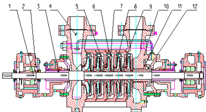
(七) AY 型多级油泵结构图
